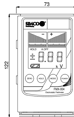
Technische tekening FMX-004
