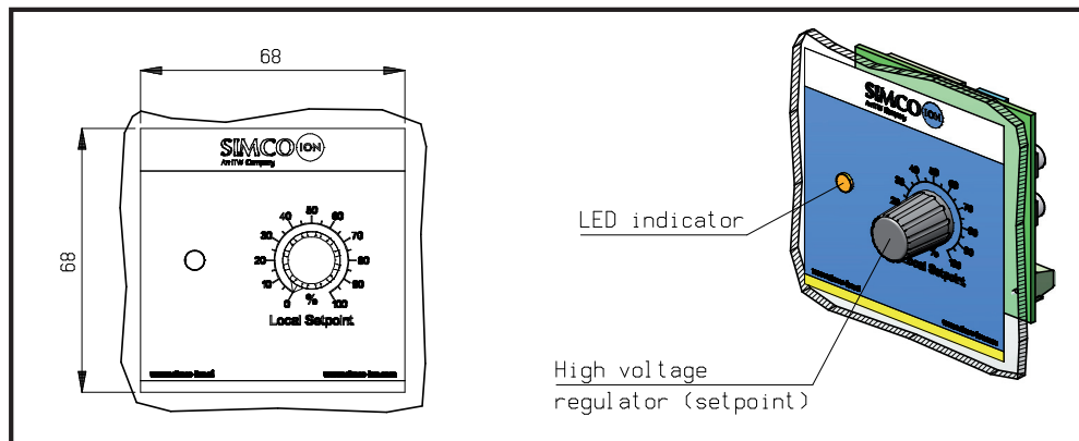
Technische tekening External balance control kit CMME/CM Tiny
