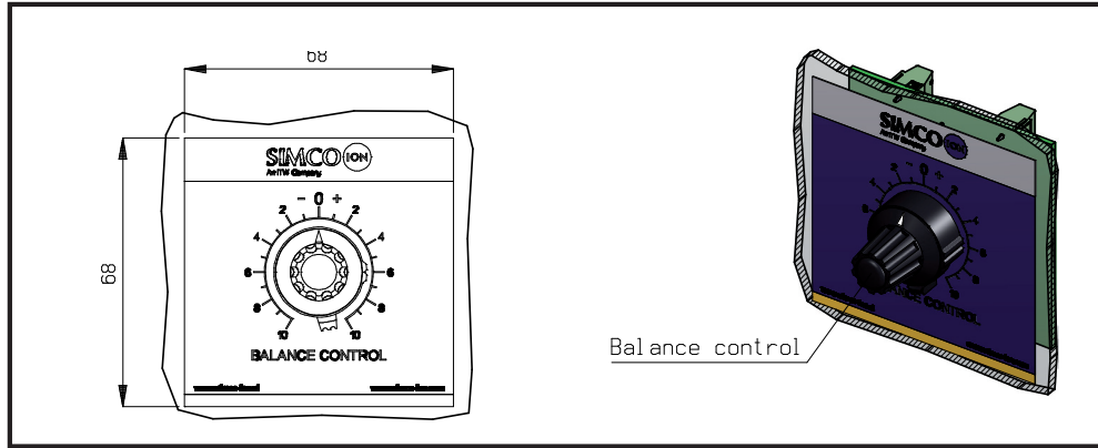
Technische tekening External control kit MPM
