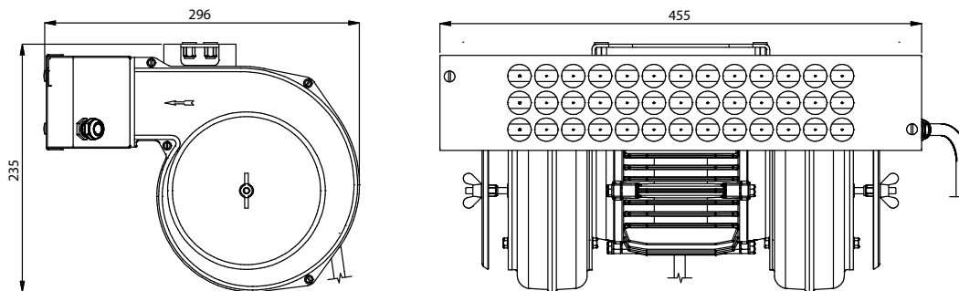
Technische tekening VolumION
